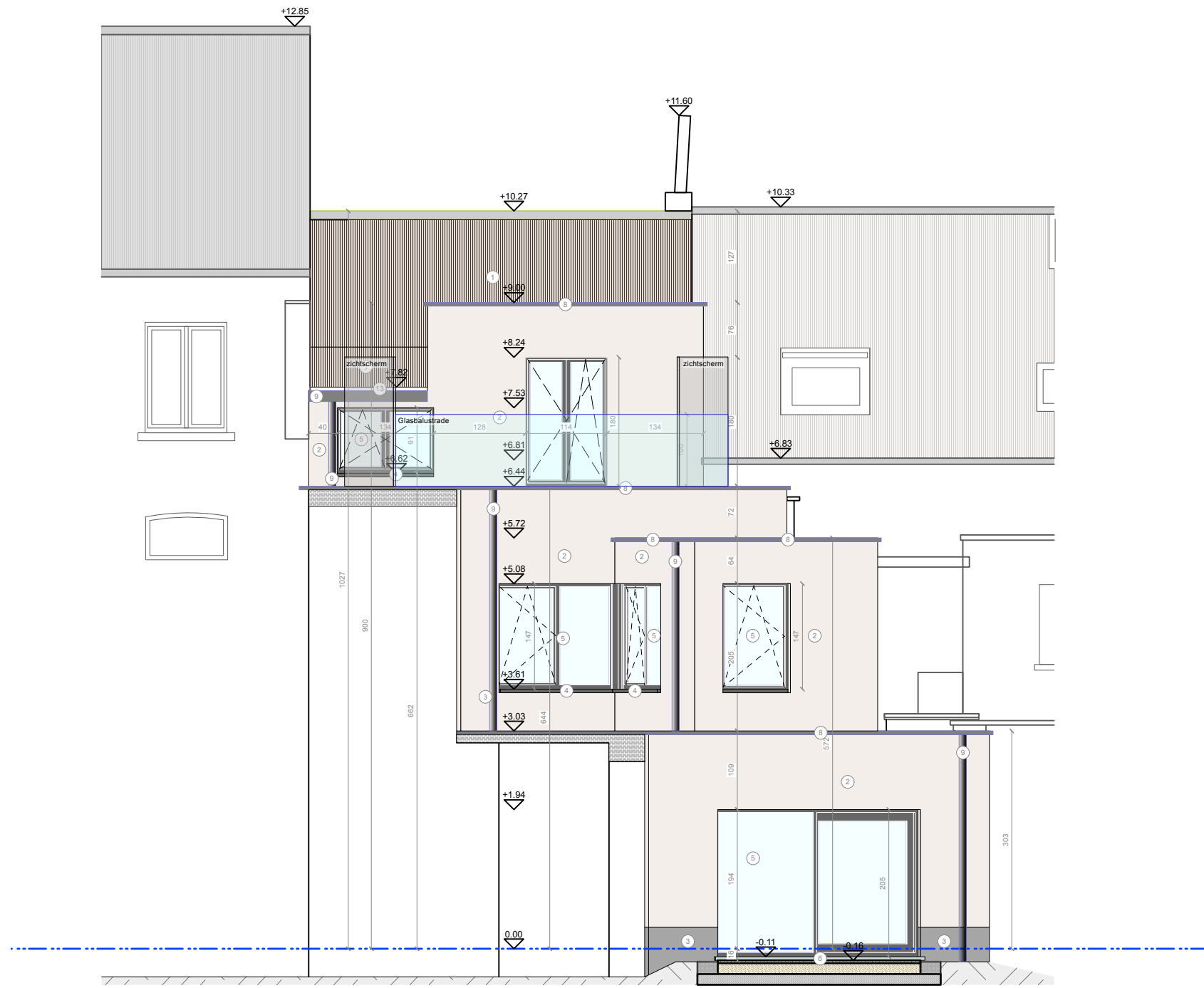
ACHTERGEVEL
